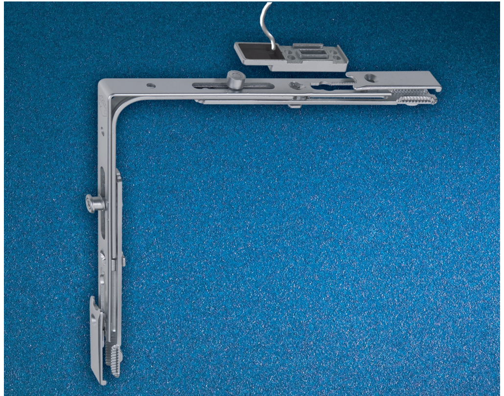
Winkeltrieb mit Sensor.
